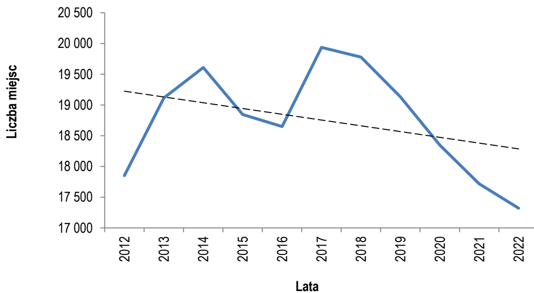
Wykres 35. Liczba miejsc w jednostkach pomocy społecznej w województwie śląskim w latach 2012-2022.
