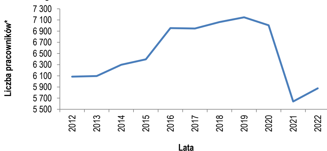
Wykres 53. Liczba pracowników* OPS / CUS w województwie śląskim w latach 2012-2022, stan na koniec danego roku.
